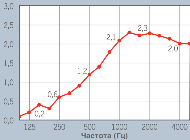
Эквивалентная поверхность звукопоглощения [м 2 ]
