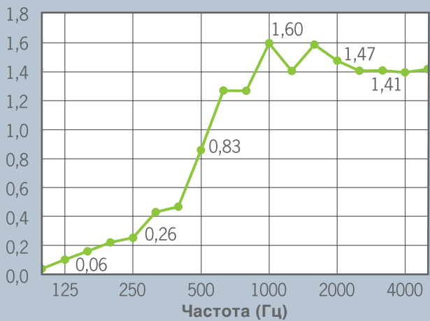
График звукопоглощения \alpha_s
